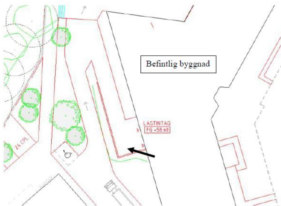
Bild. Nedfart till den befintliga byggnadens lastintag. Svart pil visar den lägsta punkten mot befintlig byggnads fasad. (Ramböll, 2024-12-23).
