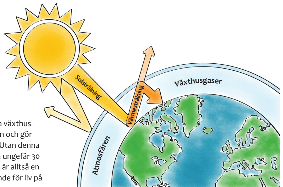
Växthuseffekten
